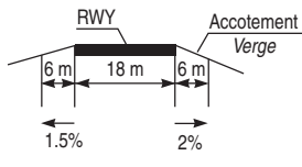
PROFIL EN TRAVERS DE LA PISTE CROSS SECTION ABEAM RWY
